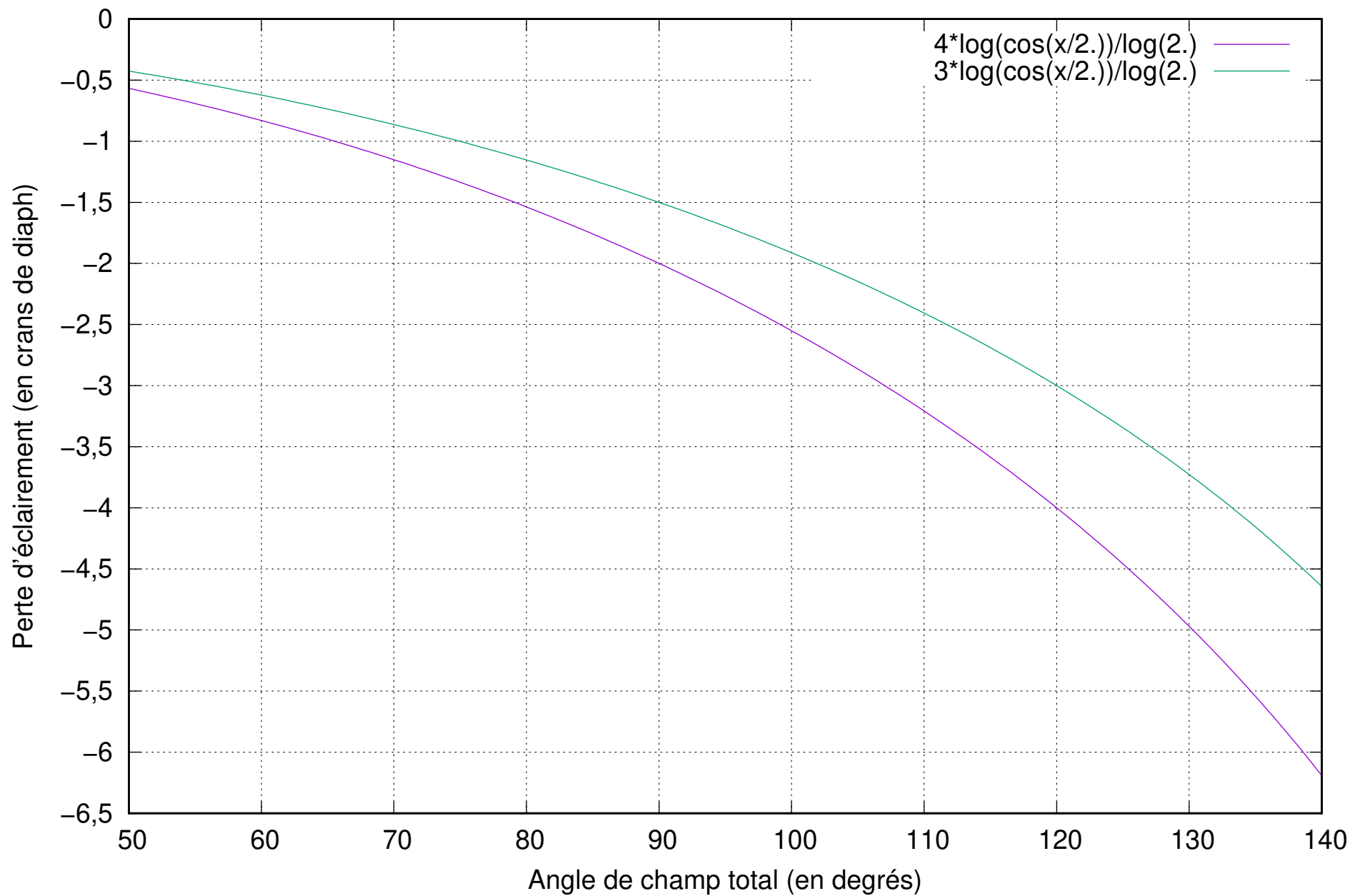
\cos^3(\theta) et \cos^4(\theta) perte d'éclairement en bord de champ, en crans de diaphs
