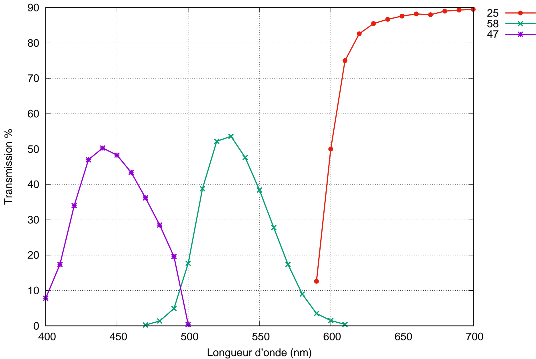
Filtres Wratten® RVB pour la trichromie directe
